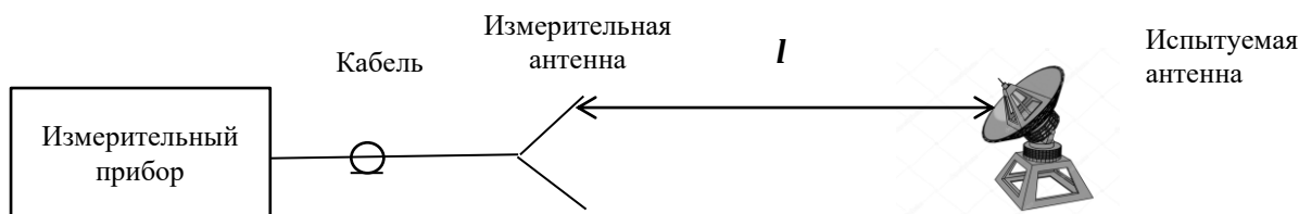
Рисунок 6 – Схема соединения приборов при измерении плотности потока энергии
