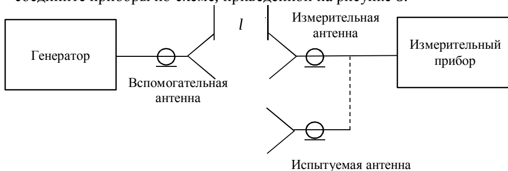
Рисунок 8 – Схема соединения приборов при измерении эффективной площади.
