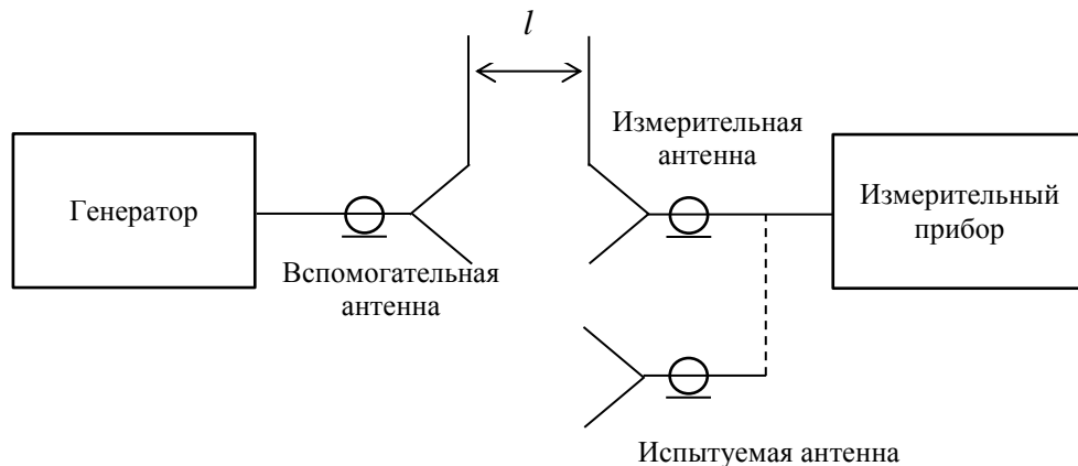
Рисунок 14 – Схема соединения приборов при измерении эффективной площади.
