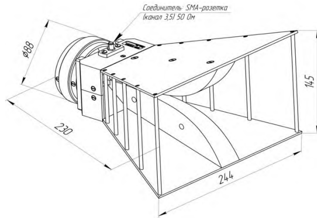
Рисунок 4 – Антенная система П6-123
