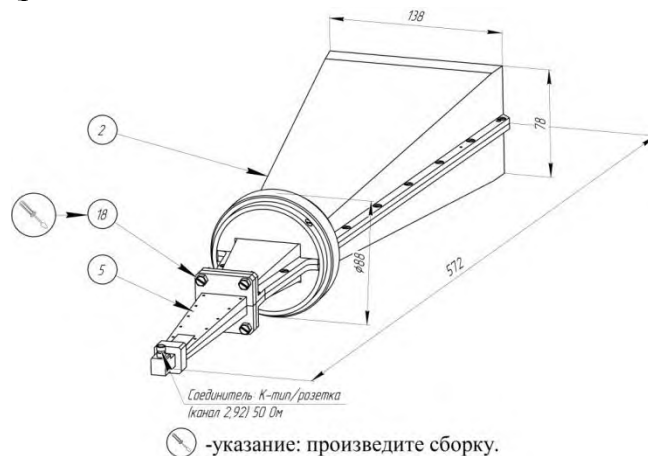
Рисунок 8 – Антенная система Пб-140-4
