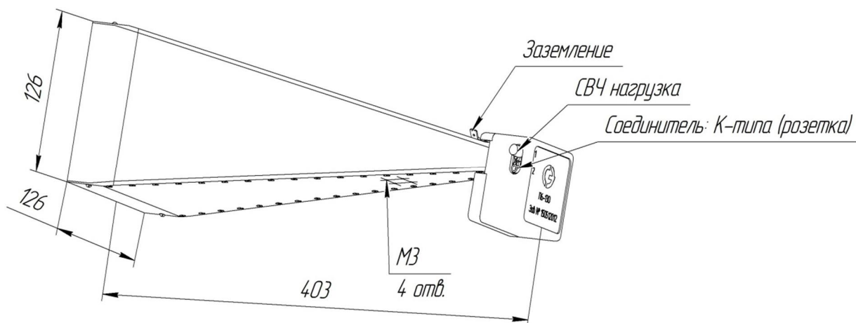
Рисунок 1 – Внешний вид рупора П6-130
