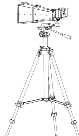
Рисунок 5 – Общий вид рупора Пб-130 в развёрнутом положении
