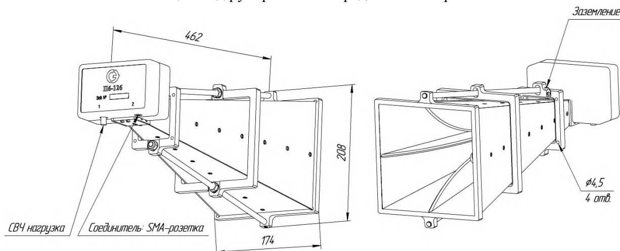
Рисунок 1 – Общий вид рупора П6-126
