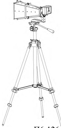
Рисунок 5 – Общий вид рупора П6-126 в развёрнутом положении.
