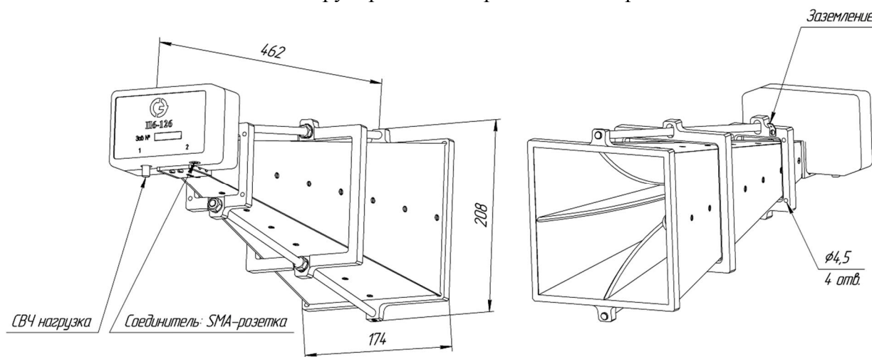
Рисунок 1 – Общий вид рупора Пб-126
