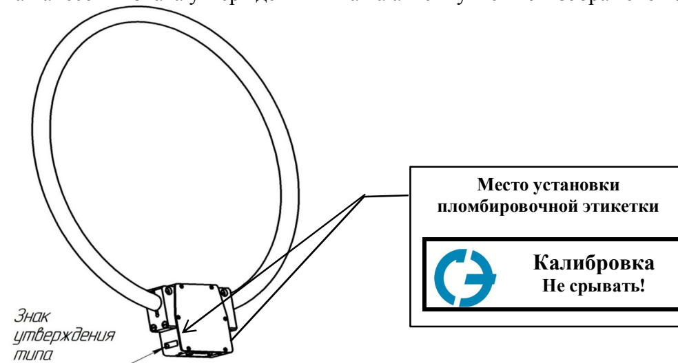
Рисунок 2 - Схема нанесения знака утверждения типа на антенну Пб-119.
