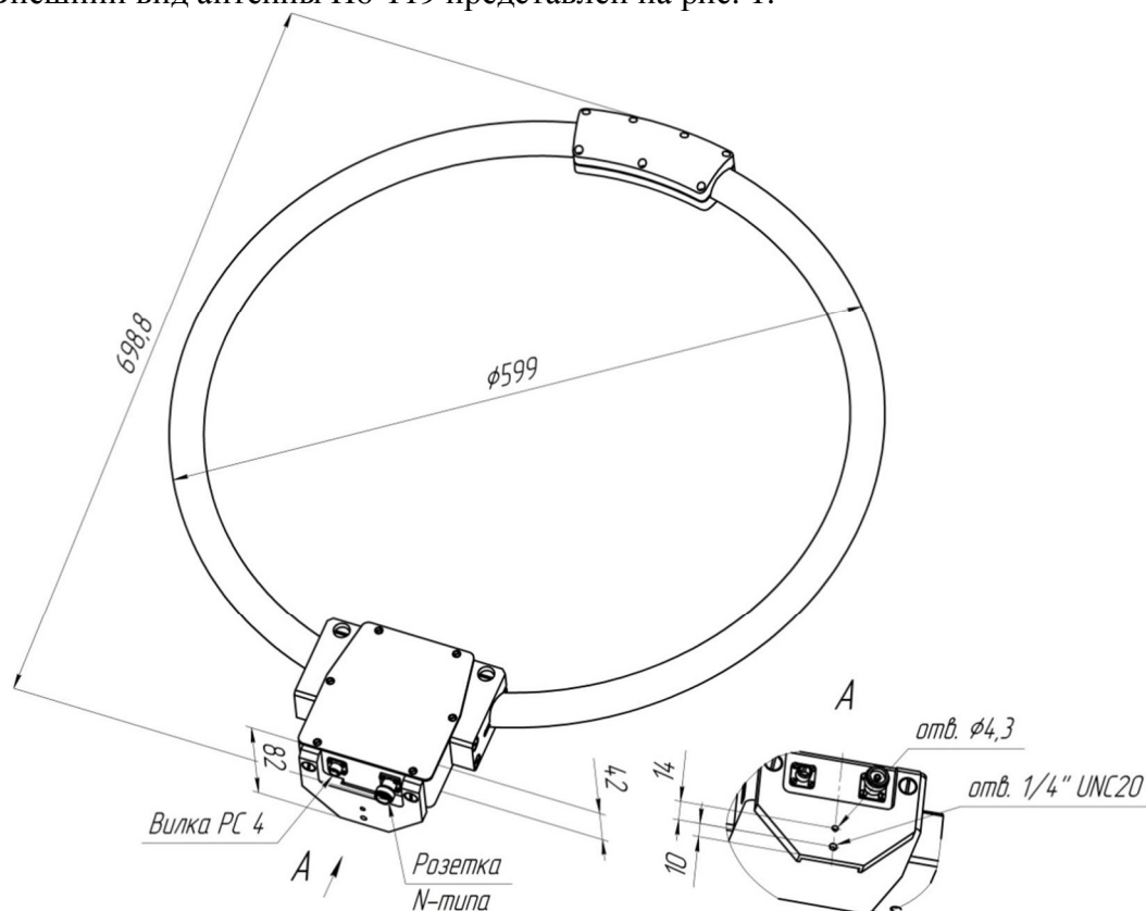
Рисунок 1 – Внешний вид антенны Пб-119
