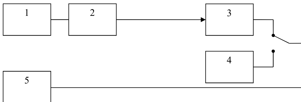
Рисунок 3 - Схема измерений коэффициента усиления антенн методом замещения
