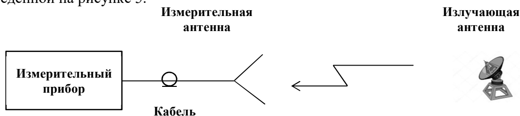
Рисунок 5 – Схема соединения приборов при измерении плотности потока энергии
