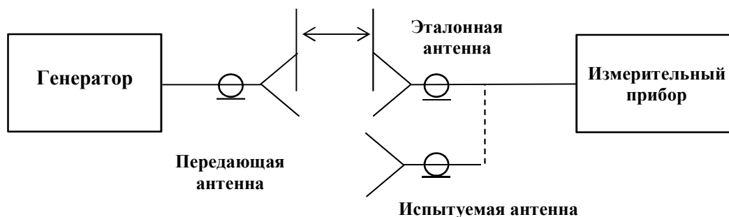
Рисунок 4 – Схема соединения приборов при измерении эффективной площади.
